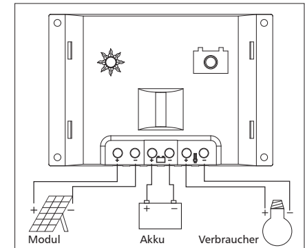
Fig. 2: Anschlussbelegung
