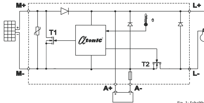
Fig. 1: Schaltbild
